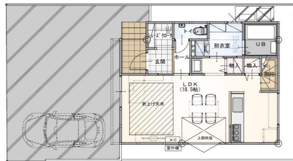
1階 平面図 S:1/100
