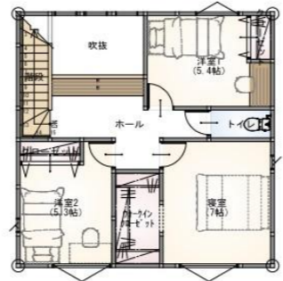
2階 平面図 S:1/100
