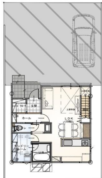
1階 平面図 S:1/100
